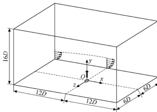
图 1 Gruber 的声速喷流试验计算域几何构型
