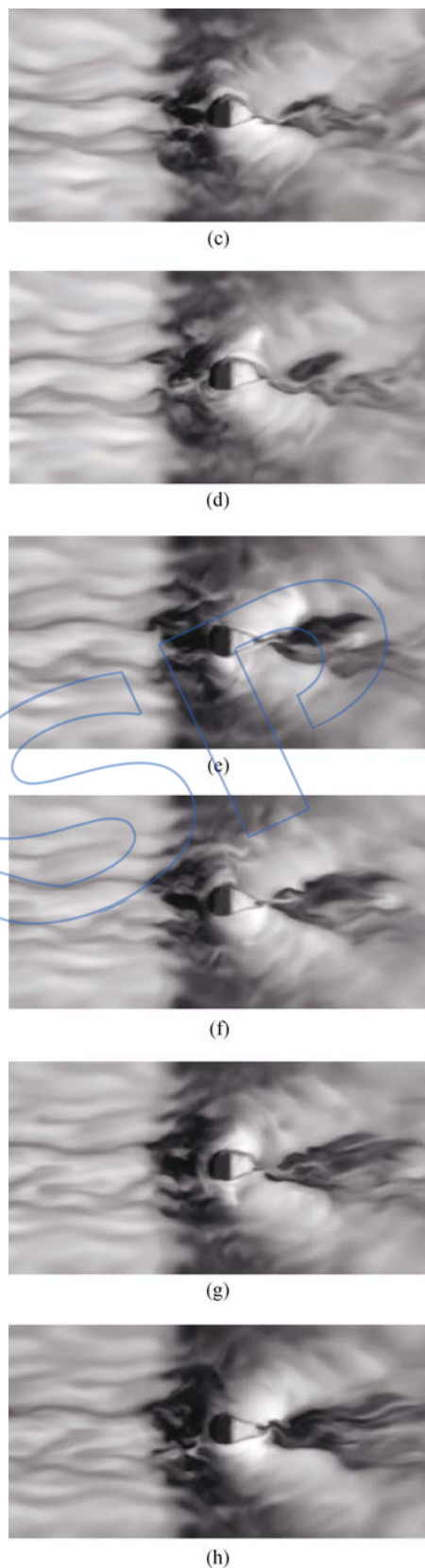
图6 x - z 中心平面上干扰区瞬时流场的流向速度云图快照
