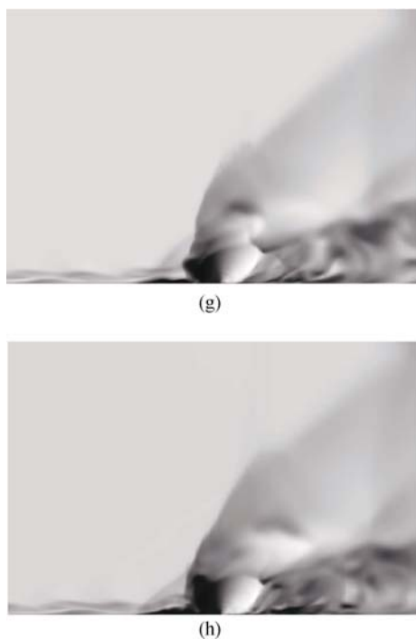
图5 x - y 中心平面上干扰区瞬时流场的流向速度云图快照
