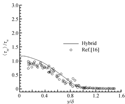
图 3 入口无量纲平均雷诺切应力分布
