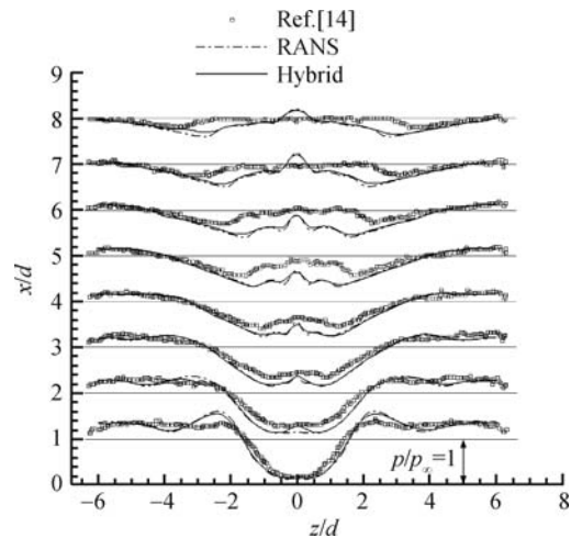
图 8 展向壁面静压分布
